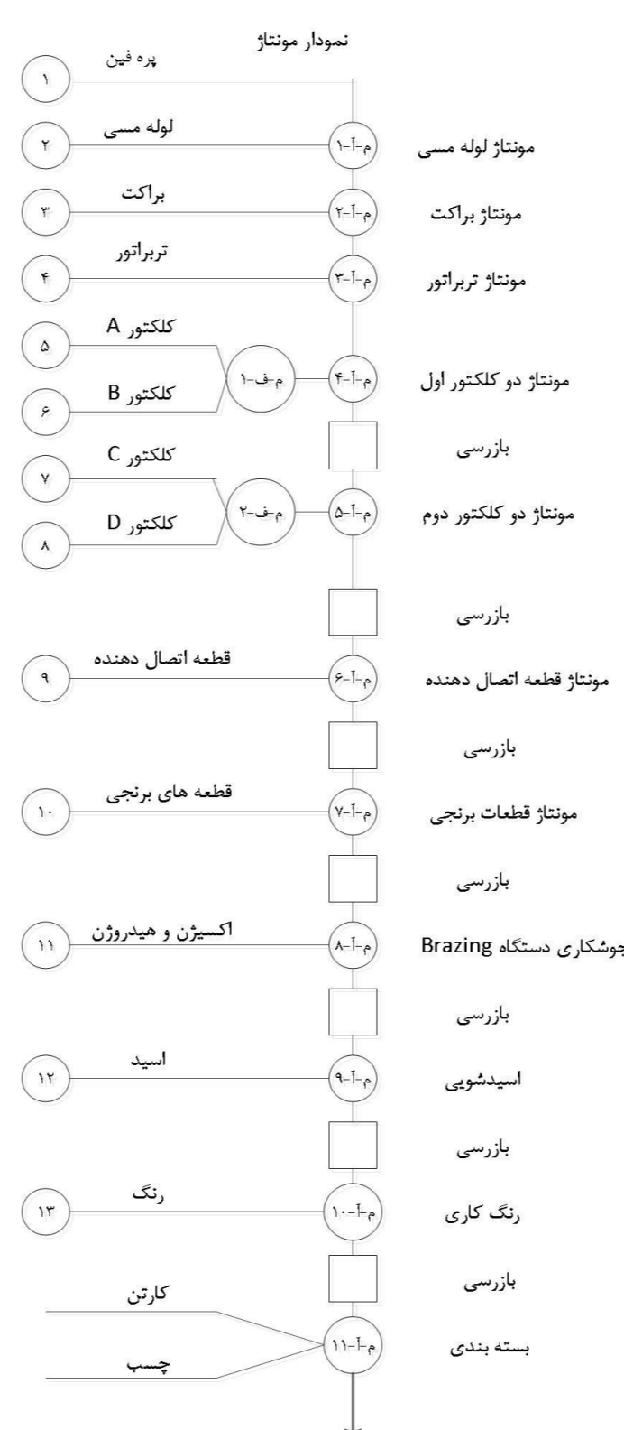
شکل 3 نمودار مونتاژ
